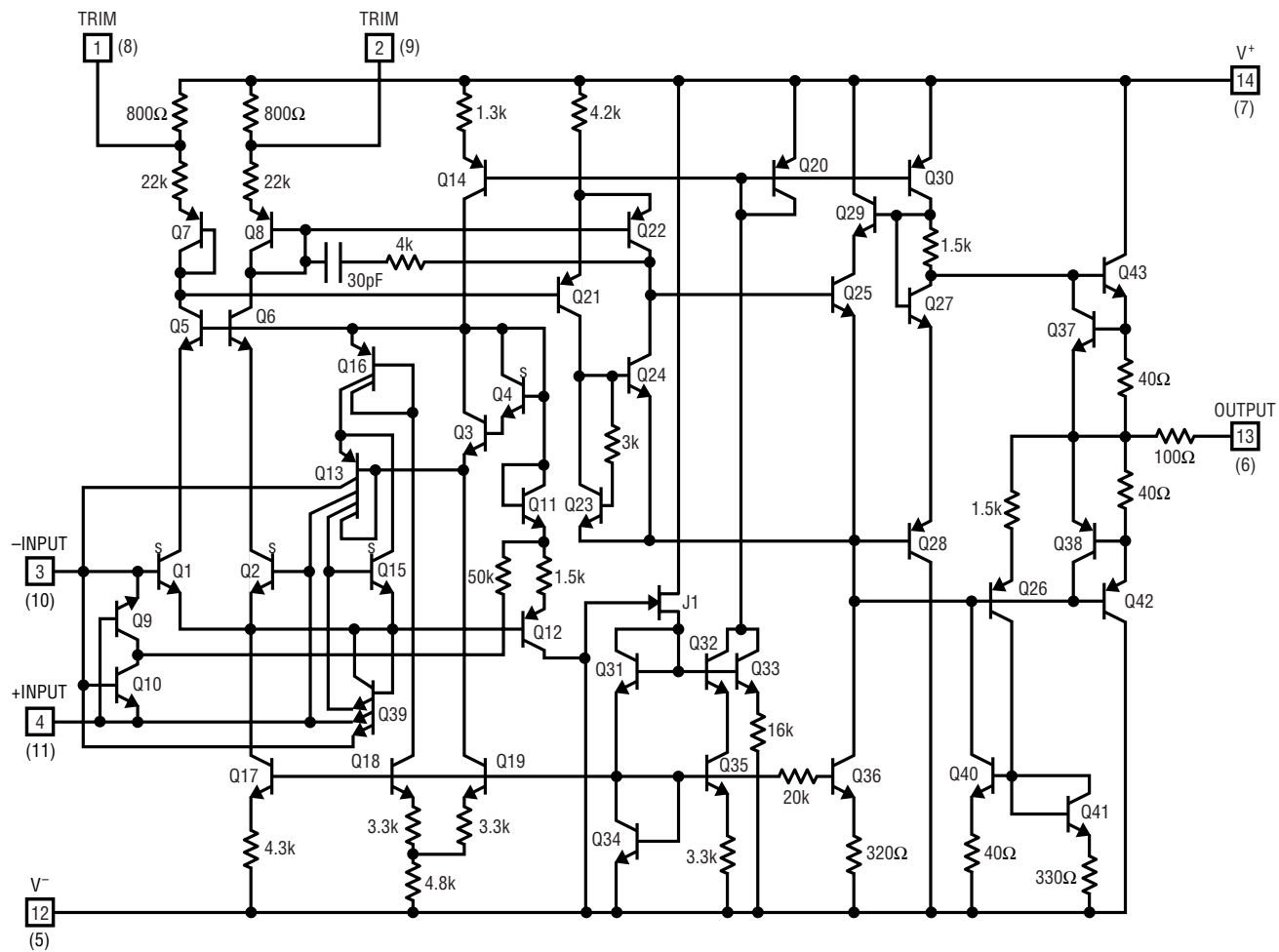
1/2 LT1024
